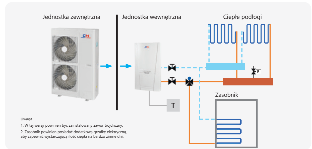
WERSJA 2 Podłączenie zbiornika wody sanitarnej
