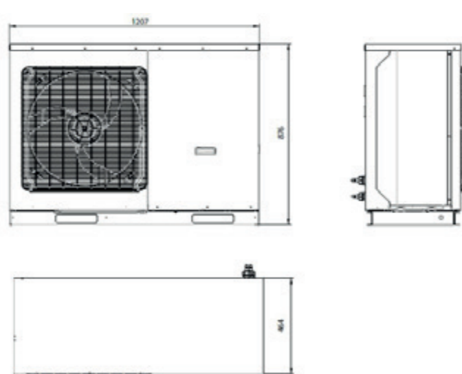
CH-HP10MIRK - CH-HP16MIRK
